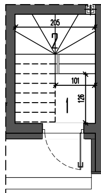
RZUT PARTERU
