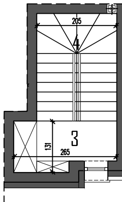
RZUT PIĘTRA
